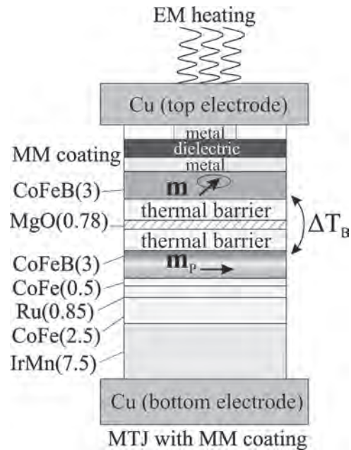
Fig.1. MTJ.
